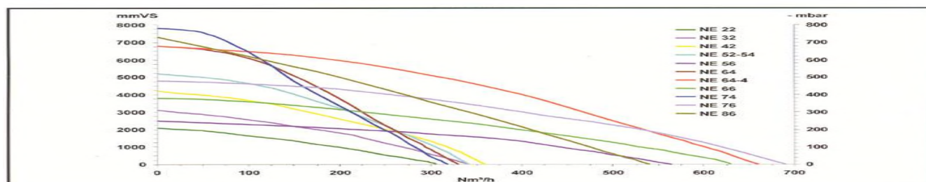
Kapasitetsdiagram (basert på trykkluft ved 7 bar)
